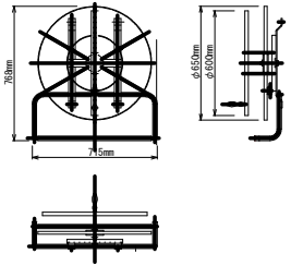
⑩ ホース巻取り機詳細図 Non Scale
