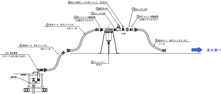
取水部 詳細図 Non Scale
